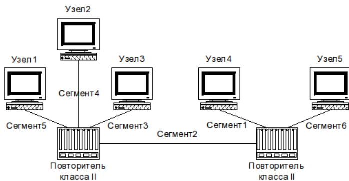
Рис. 2.3. Топология сети 2
